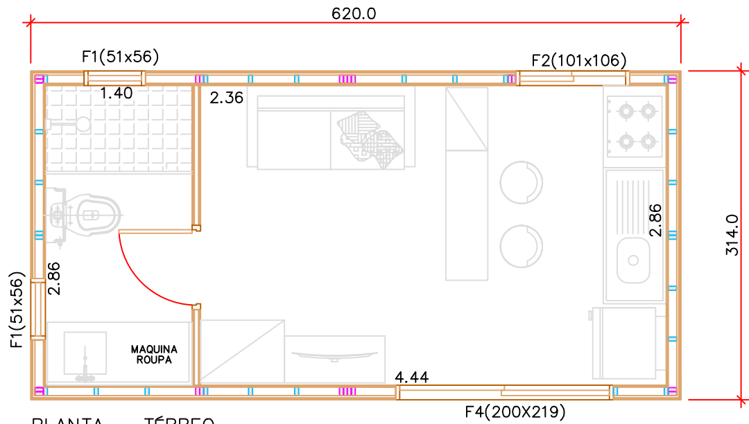
PLANTA – TÉRREO
