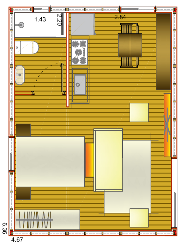
02 | Modelo 29,66 m 2 | ESC:1:50
