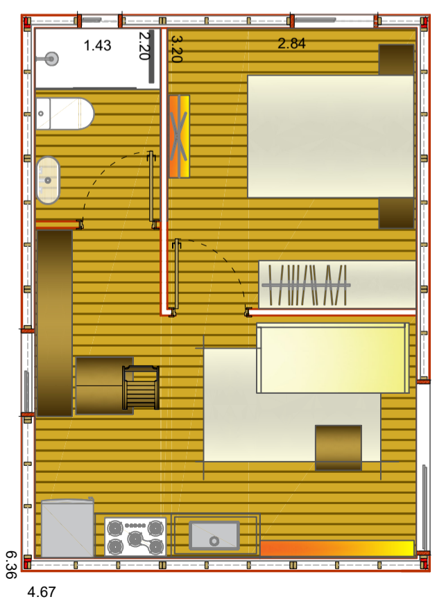
01 | Modelo 29,66 m 2 | ESC:1:50
